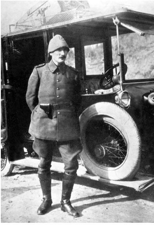
Anafartalar (1915)
